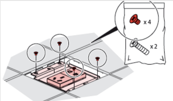
混凝土地板上（配预埋盒）
